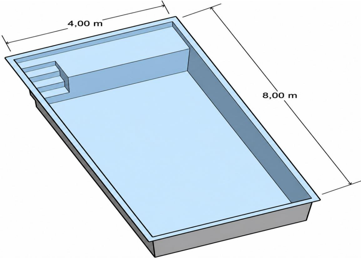
VUE 3D ISOMÉTRIQUE
