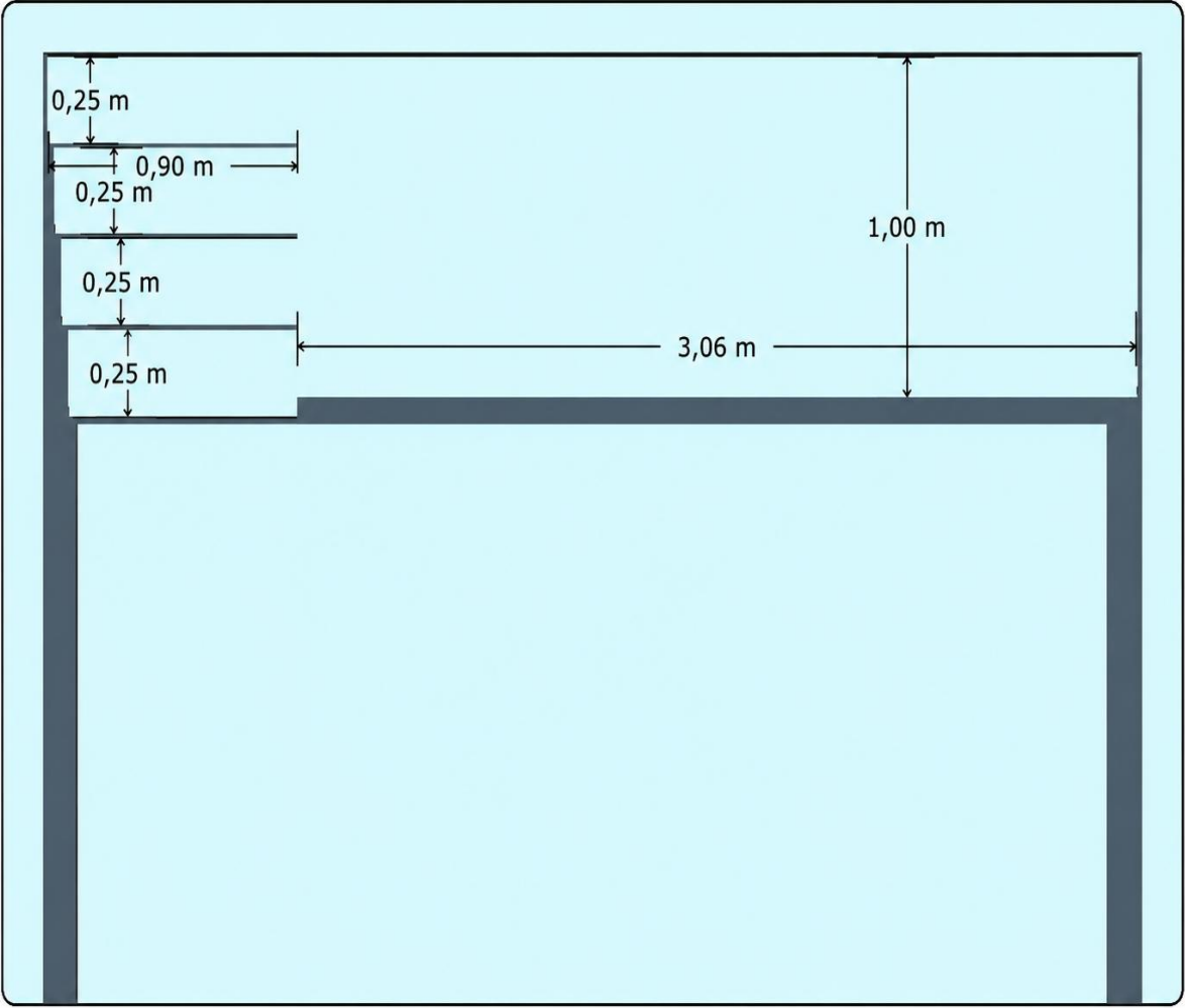
COUPE LATÉRALE (ESCALIER)
