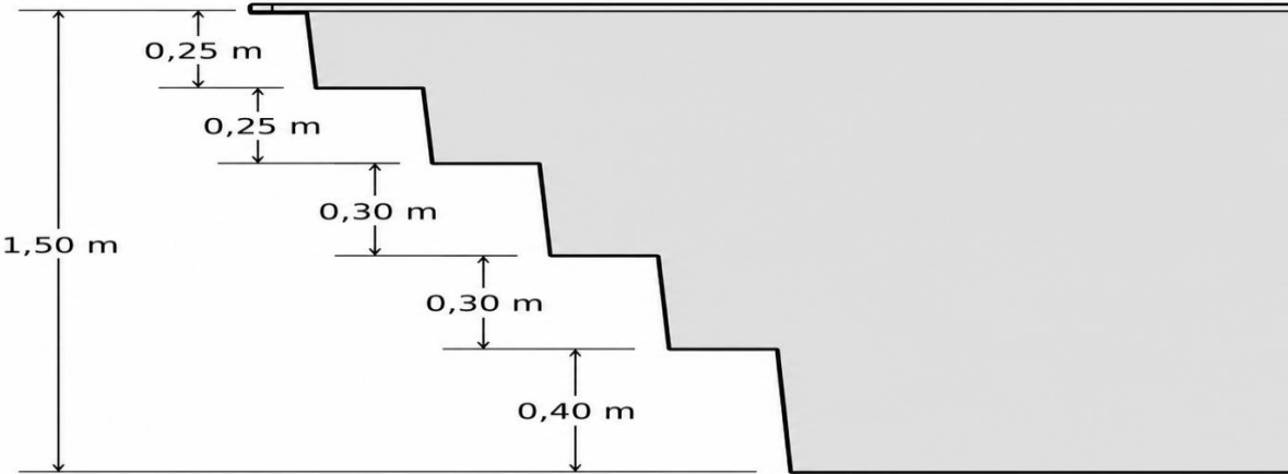
COUPE LATÉRALE (ESCALIER)
