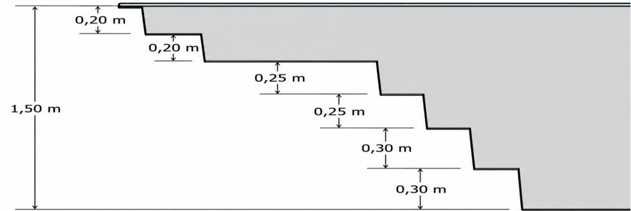
COUPE LATÉRALE (ESCALIER)
